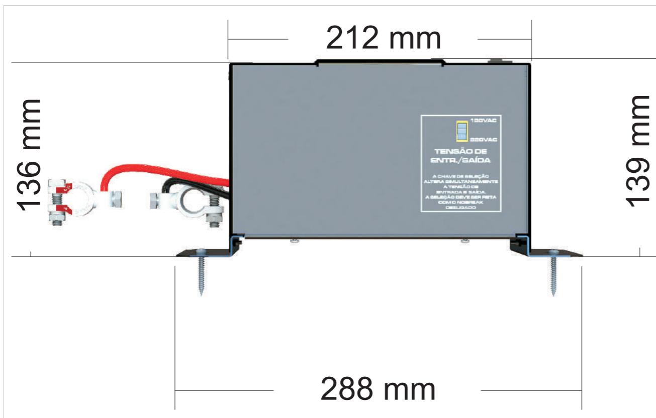
Figura 3 Dimensões - vista superior
