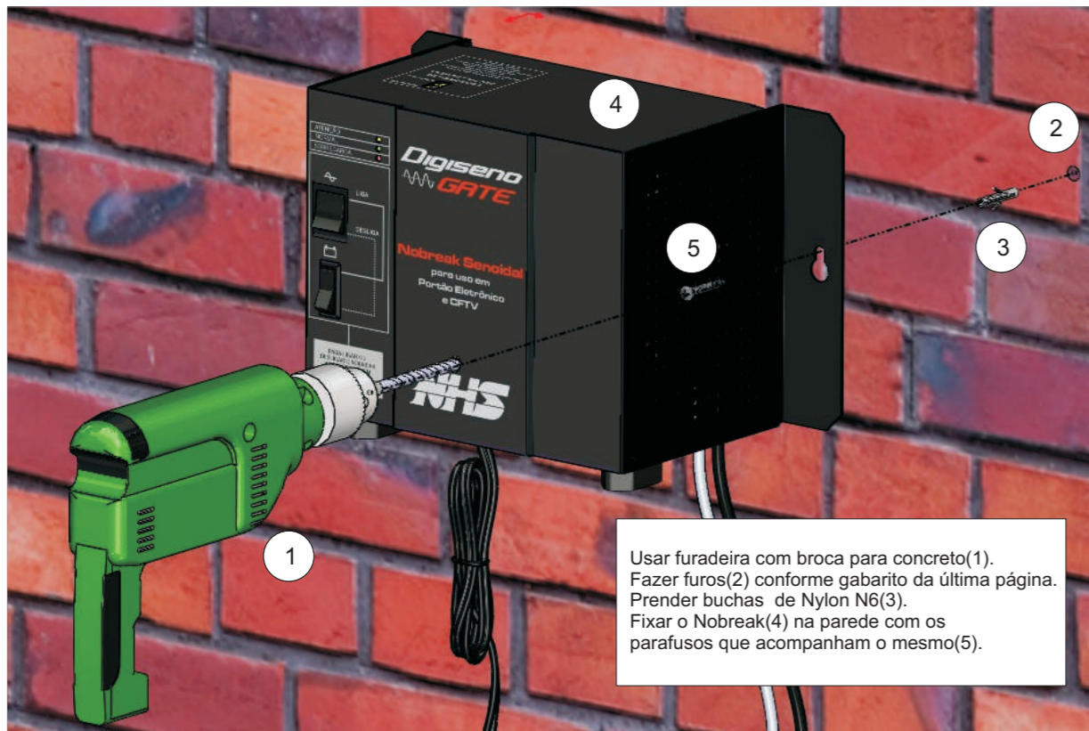
Figura 5: Exemplo de como furar a parede para fixação do Nobreak
