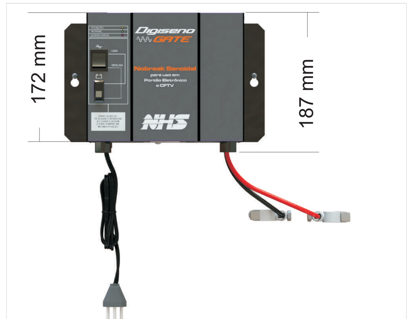
Figura 4: Dimensões - vista frontal
