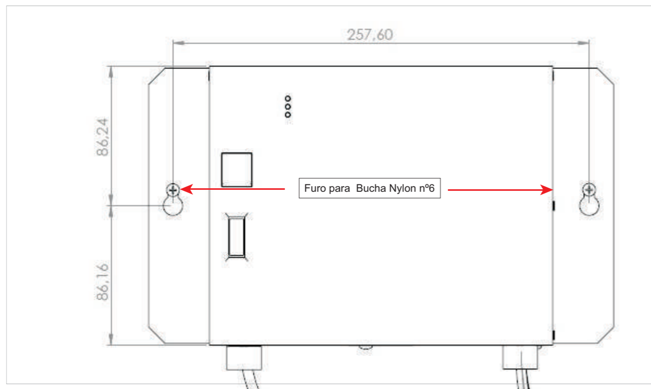
Figura 7: Diagrama de furação
