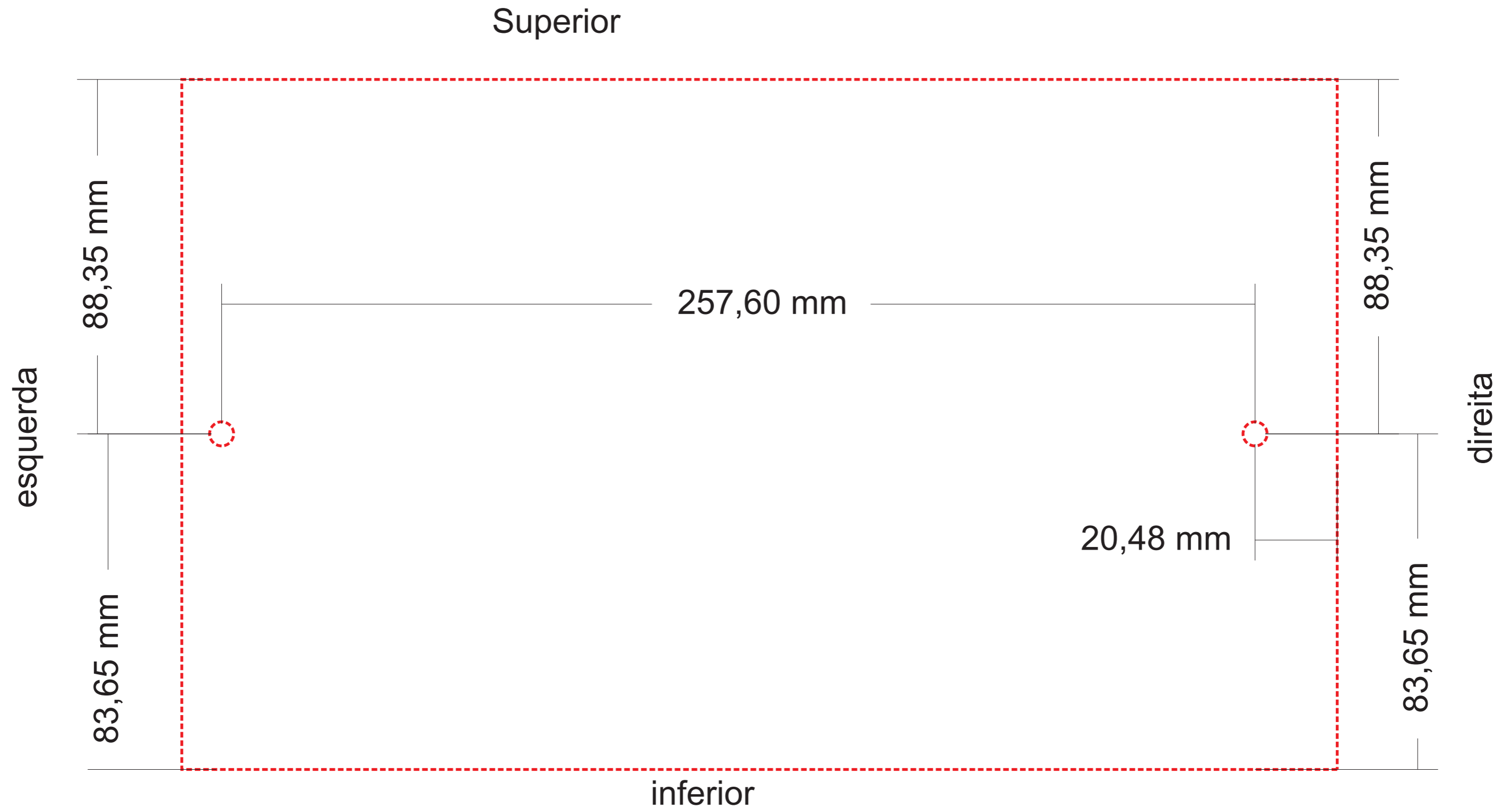
Figura 8: gabarito em escala 1:1(imprimir folha em A3).
