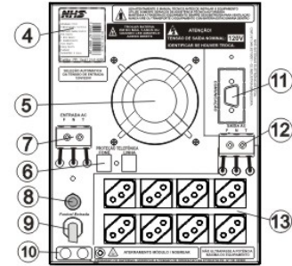
Vista traseira
